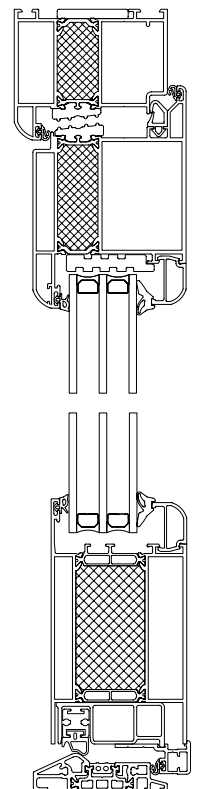
Profilschnitt senkrecht
