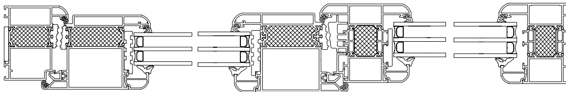
Profilschnitt waagrecht Türelement mit Seitenteil
