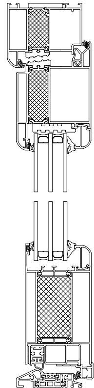
Profilschnitt senkrecht
