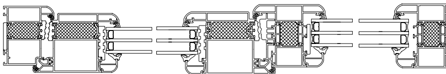
Profilschnitt waagrecht Türelement mit Seitenteil
