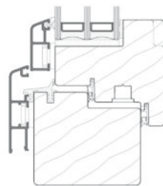
Holz-Aluminium-Fenster 82/3 flächenversetzt
