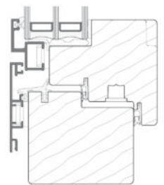
Holz-Aluminium-Fenster 82/3 flächenbündig
